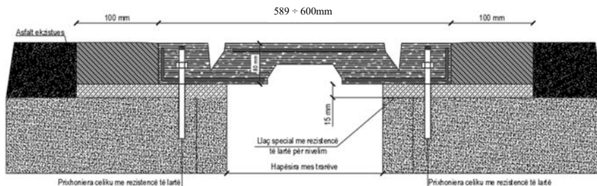
Detaj Teknik – Fuga 589 ÷ 600mm
