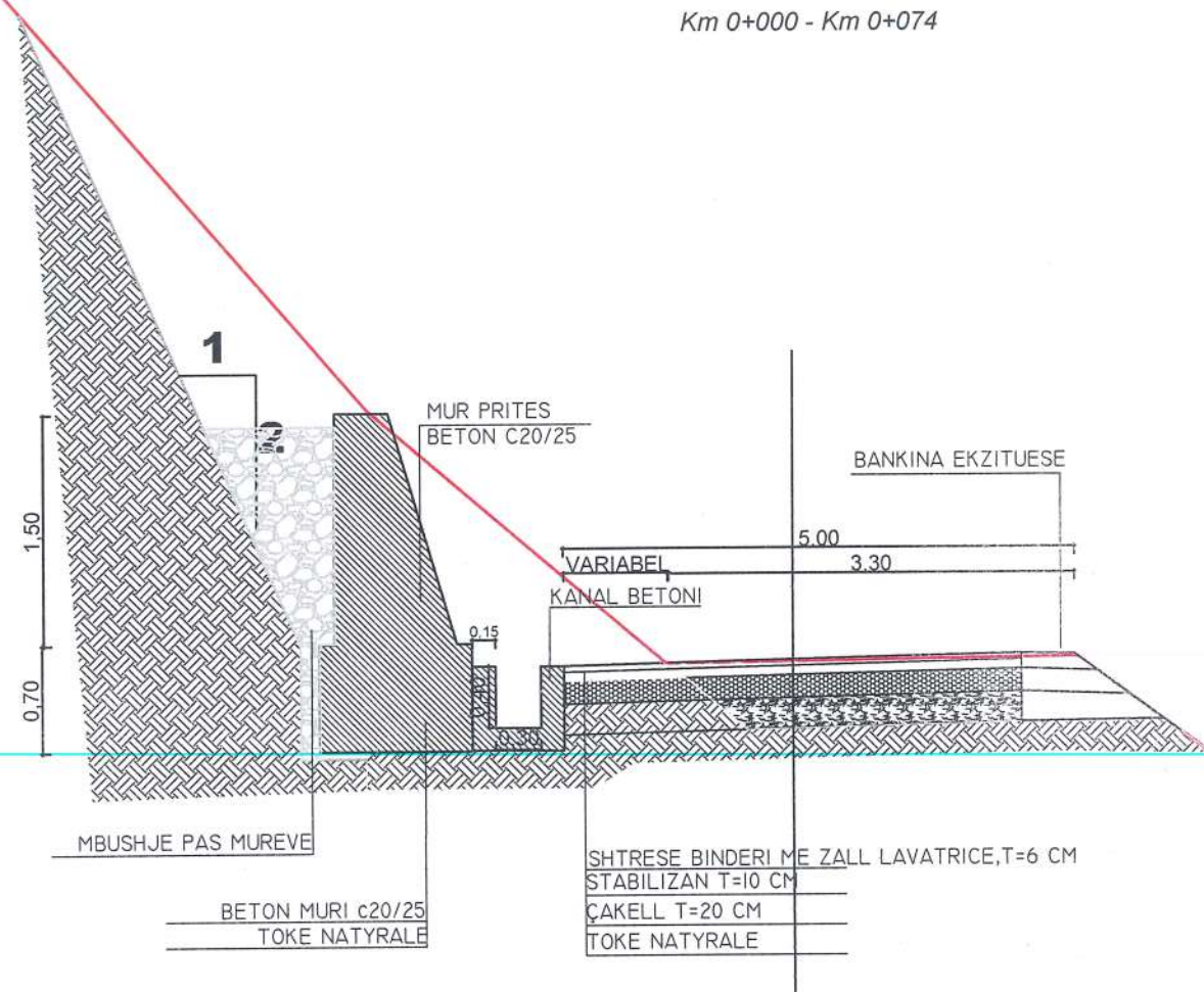
PROFIL TERTHOR TIP 1 Km 0+000 - Km 0+074
