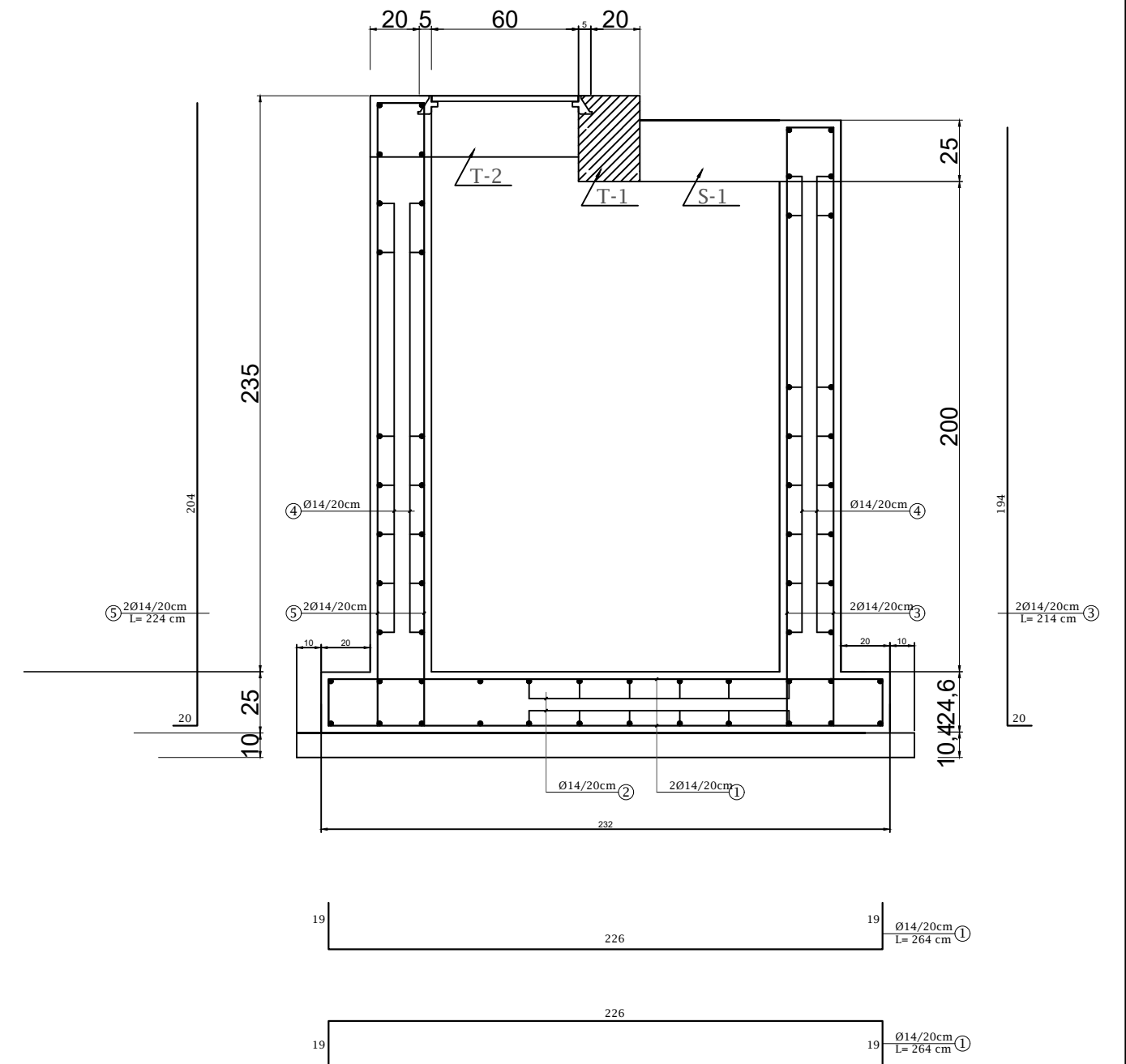
PRERJA A-A SH.1:25
